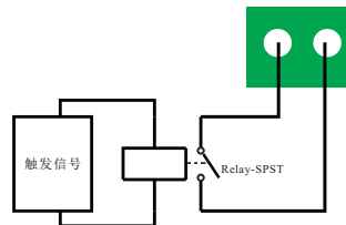
应用图2：外接继电器开关
